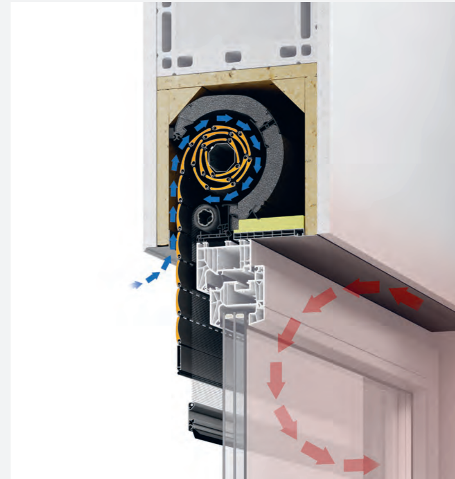
Warmluft bleibt innen, Kaltluft bleibt draußen.
