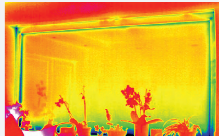
Die Wärme bleibt im Haus – Rot zeigt die perfekte Wärmedämmung nach Tausch von Fenster und Rollläden (Aufnahme von innen).
