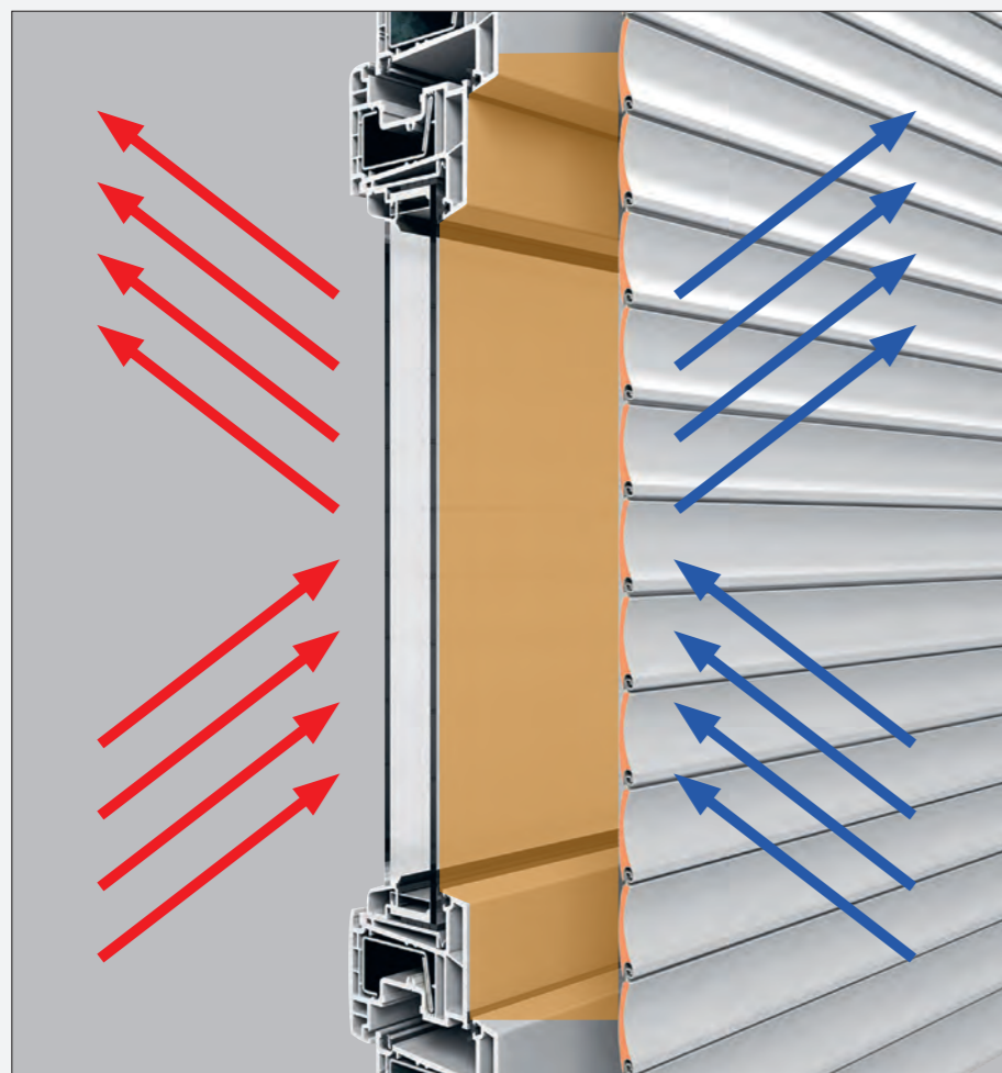
Die Luftschicht zwischen Fenster und Rollläden wirkt wärmedämmend und hilft, Heizkosten zu senken.
